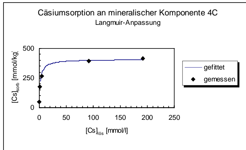
Abb. 3.21: Langmuir-Anpassung Cäsiumsorption, mineralische Komponente Etzdorf
