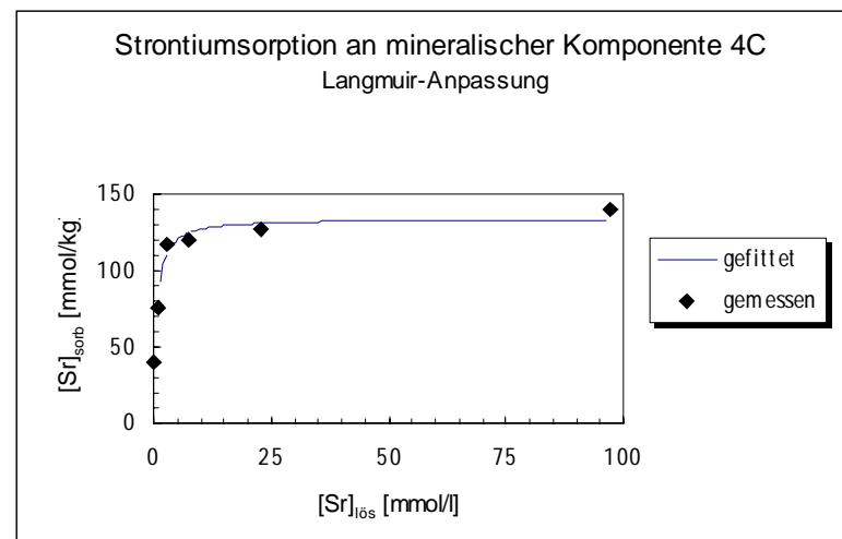
Abb. 3.30: Langmuir-Anpassung Strontiumsorption, OMK Etzdorf
