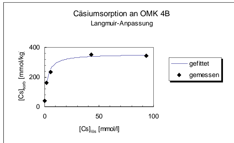
Abb. 3.20: Langmuir-Anpassung Cäsiumsorption, OMK Etzdorf
